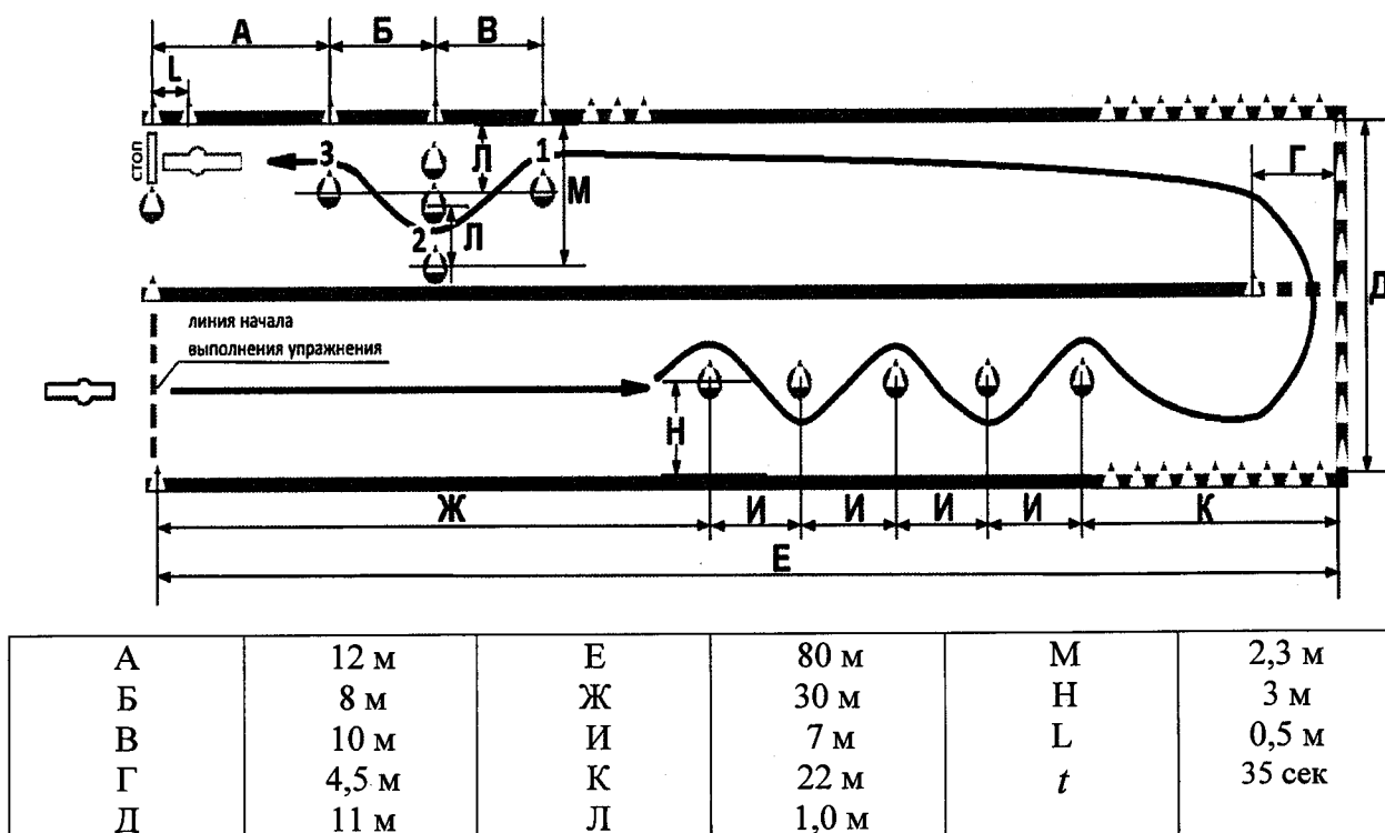
Рисунок 3. Схема и размеры элемента упражнения № 1 – «Скоростное маневрирование»
